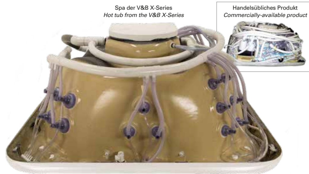
Statt veralteter Lösung mit endlosen Leitungen neue Übersichtlichkeit: kürzere Leitungen = mehr Power! Instead of outdated solutions with endless pipes, a new, streamlined layout: shorter pipes = more power!
